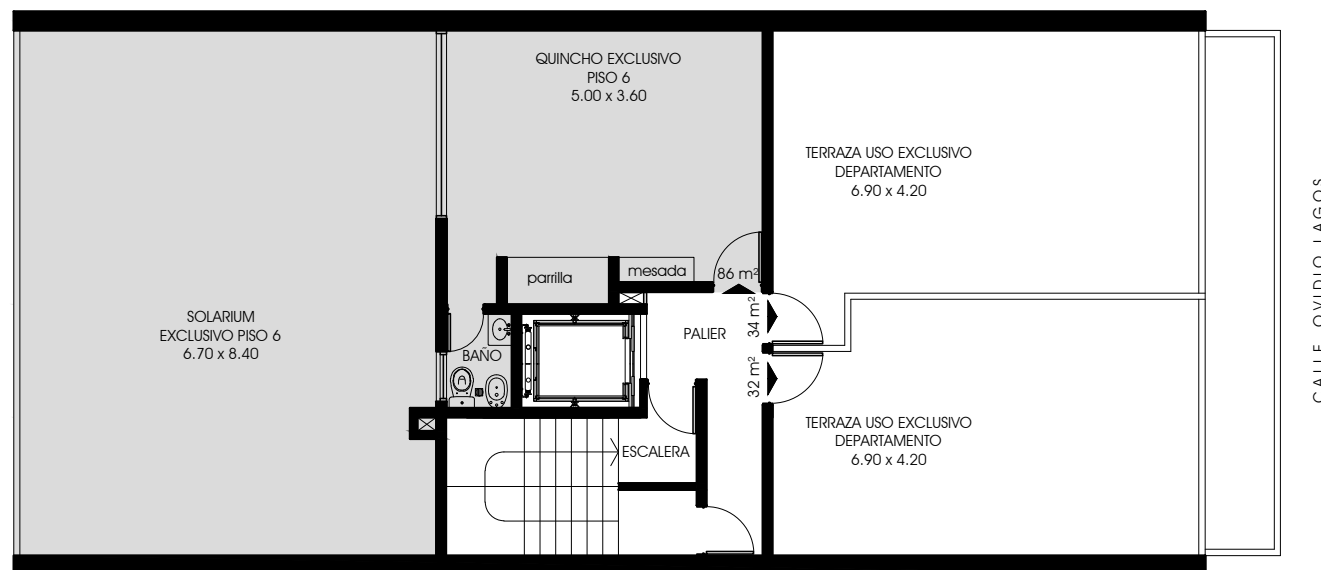
PLANTA TERRAZA
